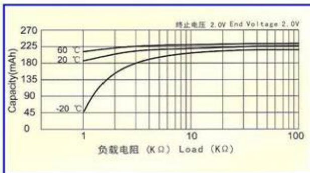
电阻容量曲线 Load-capacity
